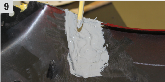
Repaplast Repair (2K-Kunststoffkleber) auf der Innenseite der Schadstelle auftragen.
