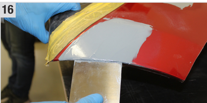
16 Das vermischte Repaplast Finish (2K-Kunststoffkitt) verspachteln und ca. 20 Min. trocknen lassen.
