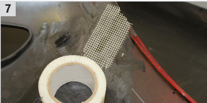
Einen Streifen Drywall Tape (Selbstklebendes Glasfasergewebeband) zuschneiden und auf der Rückseite entsprechend anbringen.
